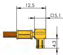
MCX-m (angular 90°)*
